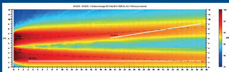
AH4335 mit 2 unabhängigen Strahlen und 2 Hörbereichen
