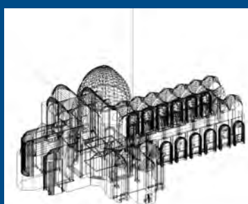
EASE-Simulation: STI-Index-Vorhersage mit zwei Ascolto LH6425 über dem Hörbereich (Kirchenschiff)
