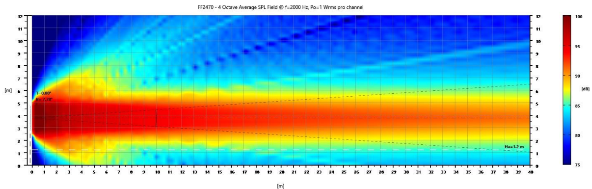
FF2470 – Vertikales Strahlmuster bei 2000 Hz, 4 Oktaven Durchschnitt
