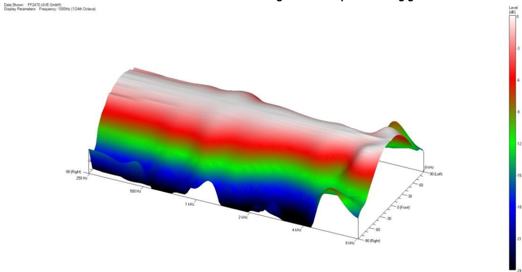
FF2470 – 3D horizontaler Öffnungswinkel frequenzabhängig
