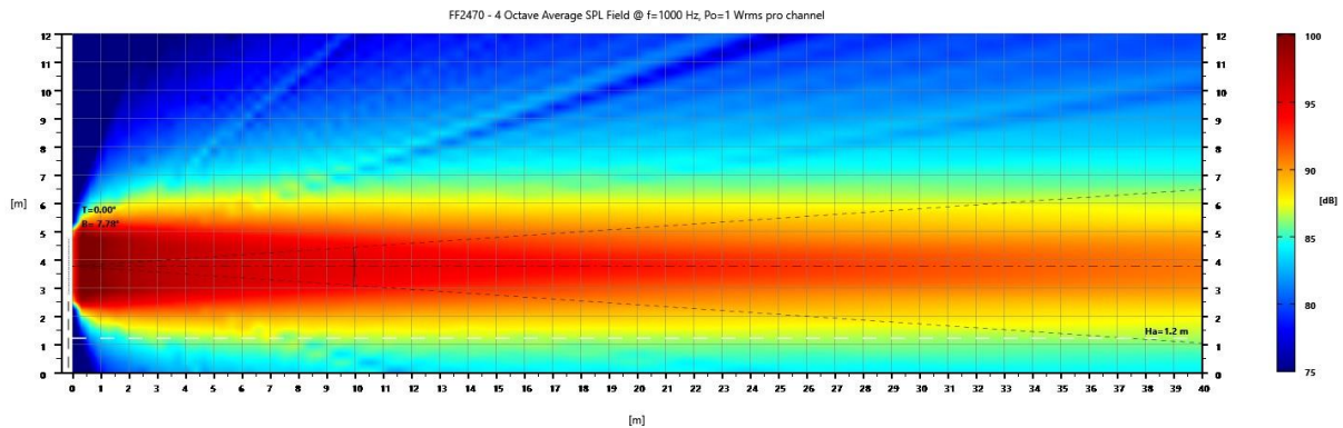
FF2470 – Vertikales Strahlmuster bei 1000 Hz, 4 Oktaven Durchschnitt
