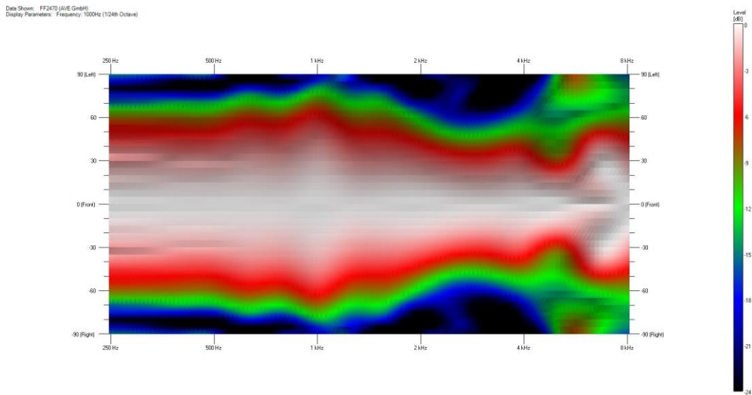
FF2470 – 2D horizontaler Öffnungswinkel frequenzabhängig
