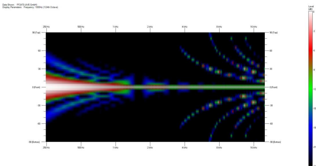
FF2470 – 2D Vertikaler Öffnungswinkel frequenzabhängig
