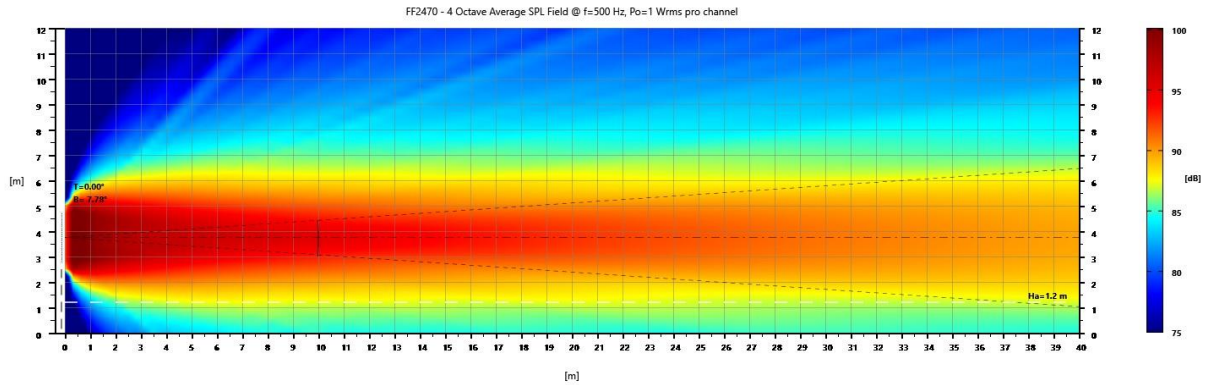
FF2470 – Vertikales Strahlmuster bei 500 Hz, 4 Oktaven Durchschnitt
