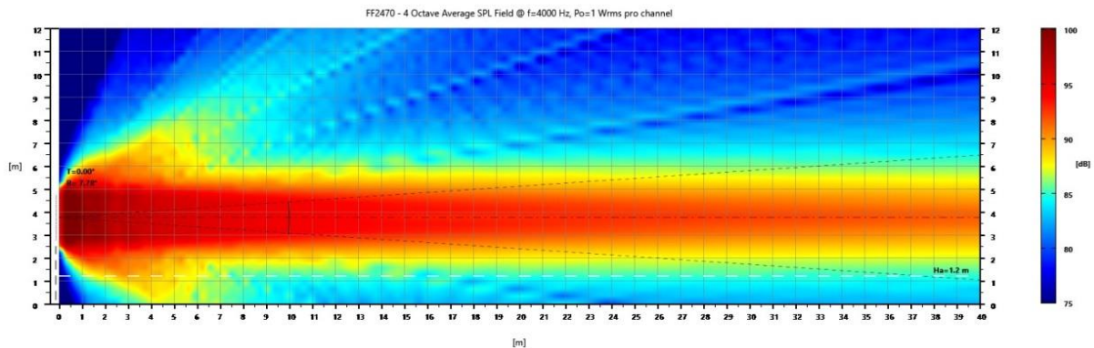
FF2470 – Vertikales Strahlmuster bei 4000 Hz, 4 Oktaven Durchschnitt
