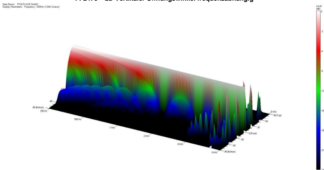
FF2470 3D Vertikaler Öffnungswinkel frequenzabhängig
