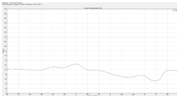
FF2470 – 3D Horizontaler Öffnungswinkel frequenzabhängig
