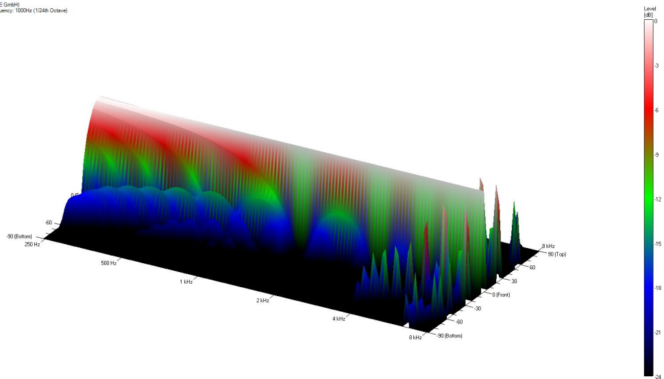
FF2470 - 3D Vertikaler Öffnungswinkel frequenzabhängig
