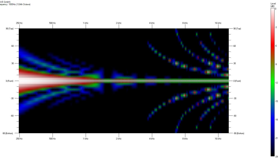
FF2470 – 2D Vertikaler Öffnungswinkel frequenzabhängig
