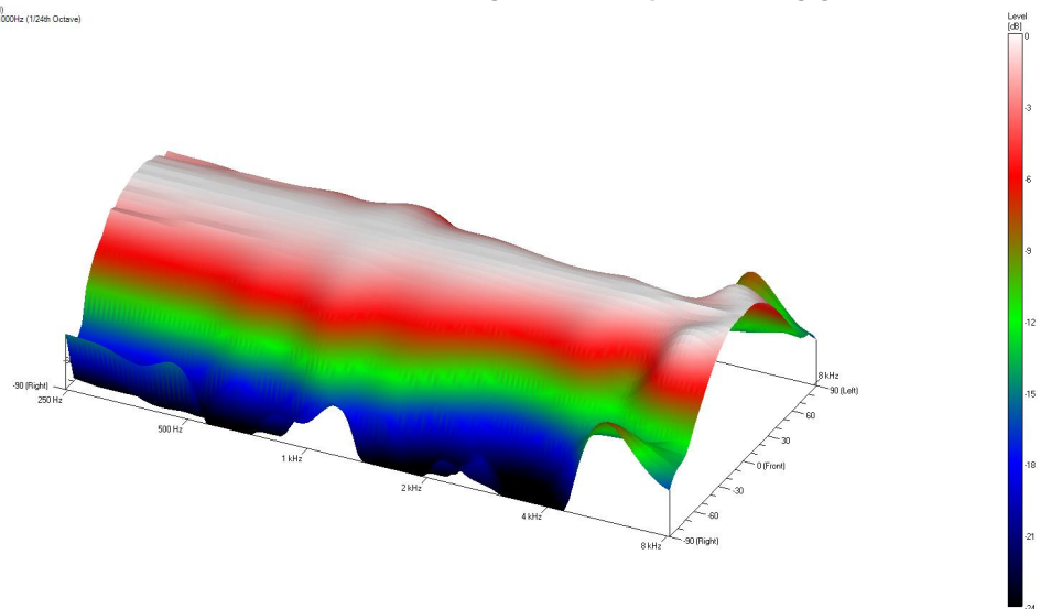
FF2470 – 3D Horizontaler Öffnungswinkel frequenzabhängig
