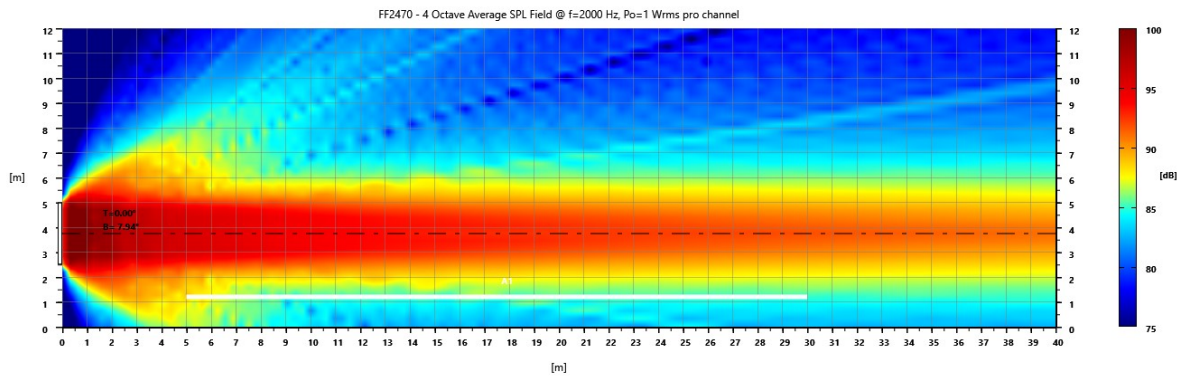
FF2470 – Vertikales Strahlmuster bei 2000 Hz, 4 Oktaven Durchschnitt
